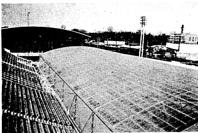
おなじみの神宮プールに屋根が設けられ一応臨時の室内プールとなって、強化合宿に大きな貢献をした。 (昭和38年12月末竣功)
